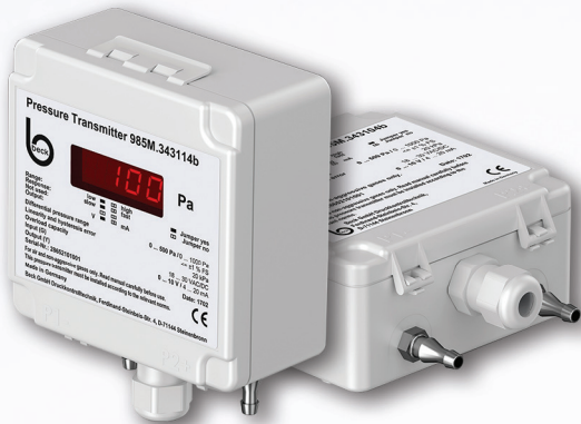
משדר לחץ הפרשי
